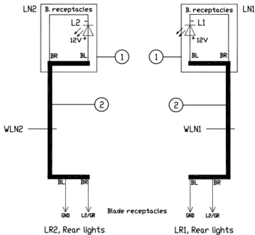
Elkretsschema registreringsskyltbelysning
