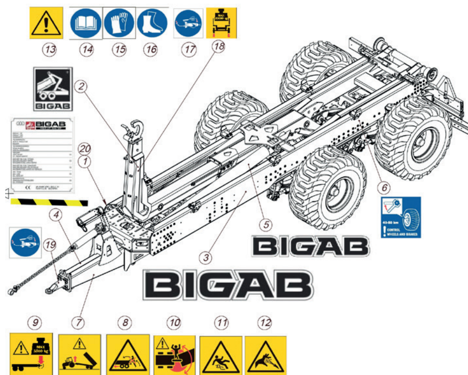
Dekalernas placering
